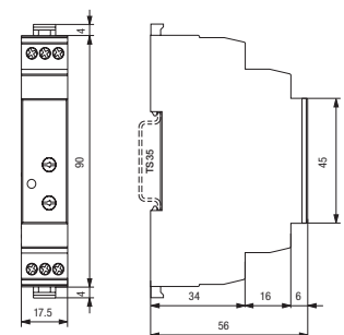
fig. 4. dimensions (mm)
