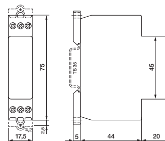
fig. 4. Dimensions (mm)
