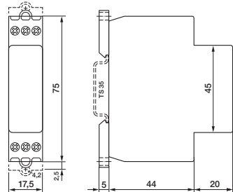
fig. 4. dimensions (mm)
