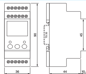
fig. 4. Dimensions (mm)
