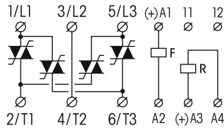
fig. 1. Wiring diagram
