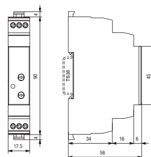
fig. 4. dimensions (mm)
