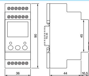
fig. 4. Dimensions (mm)
