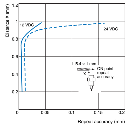
E2E-C05S01□
