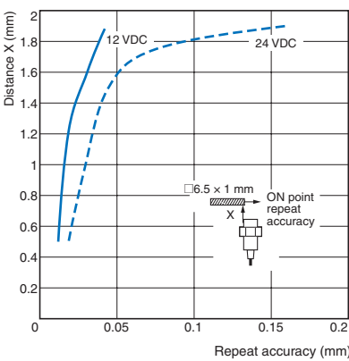
E2E-C06S02□
