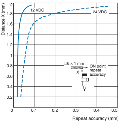
E2E-C03N02□/E2E-S04N02□
