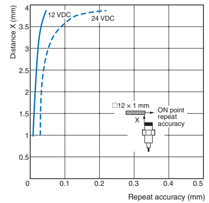
E2E-C06N04□
